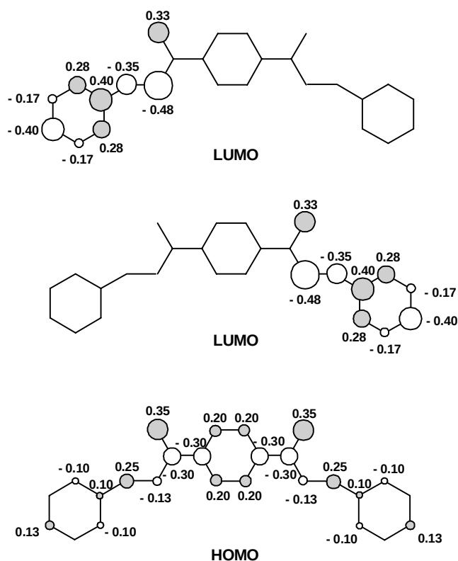
Abb. 4 Grenzorbitale (HMO-Rechnung) von 3-Phenyl-1-[4-(3-phenylpropenoyl)phenyl]prop-2-en-1-on ( 2e' )
