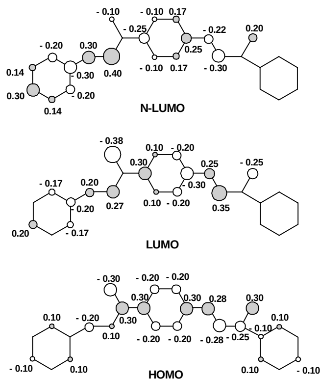
Abb. 2 Grenzorbitale (HMO-Rechnung) von 1-Phenyl-3-[4-(3-phenylpropenoyl)phenyl]prop-2-en-1-on ( 1e )
